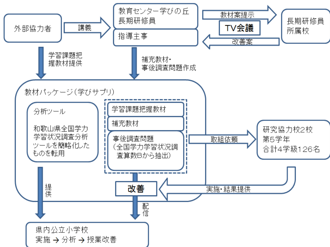
図 1 研究構想図
